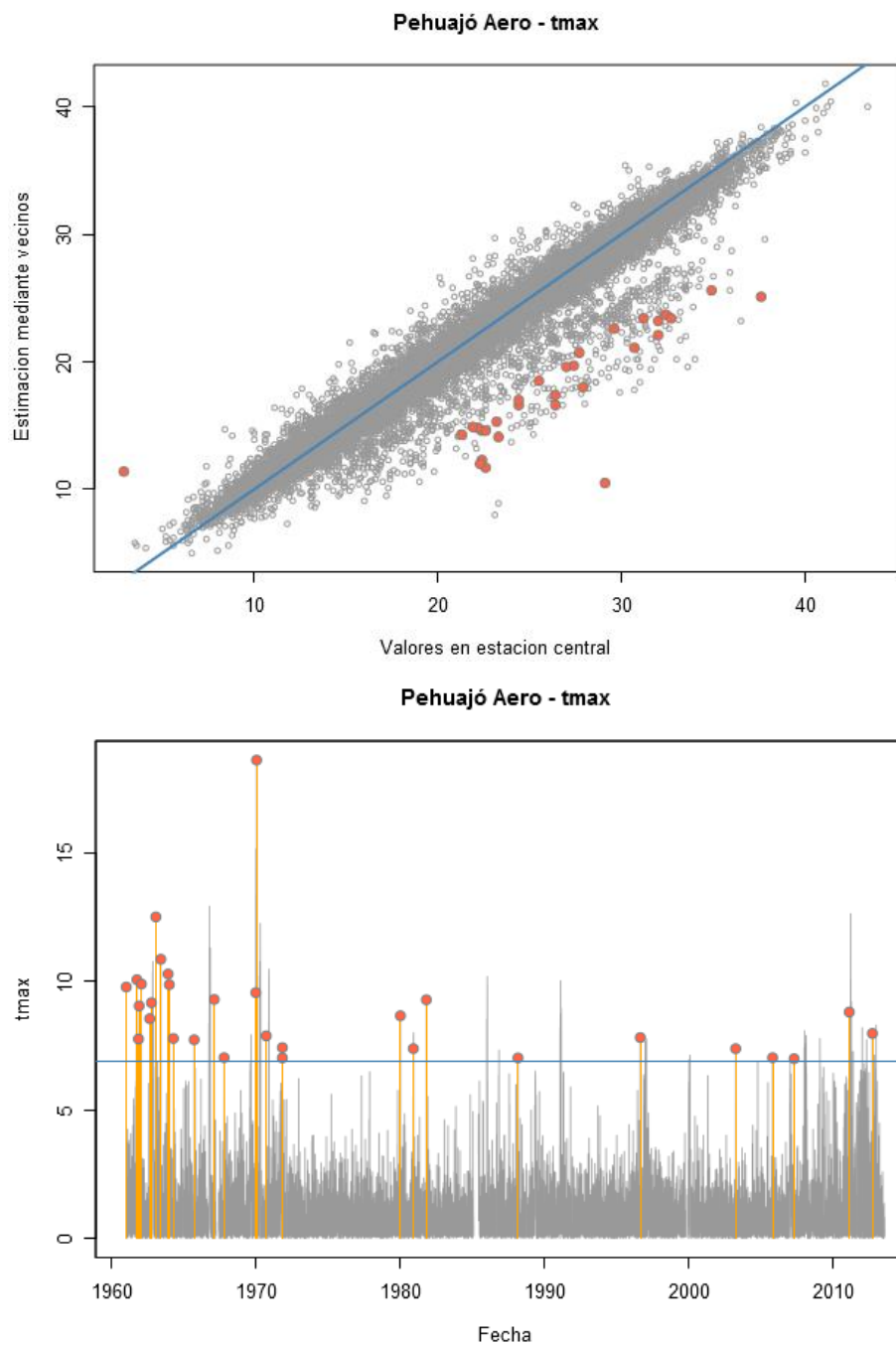
Figura 29. Panel superior: relación entre los valores observados de temperatura máxima en Pehuajó, Argentina y los valores estimados en base a 4 estaciones vecinas. Los puntos identificados como sospechosos se muestran en rojo y la línea 1:1 en azul. Panel inferior: Serie temporal de residuos para la estación central. El umbral para la identificación de valores sospechosos es la línea horizontal azul.
