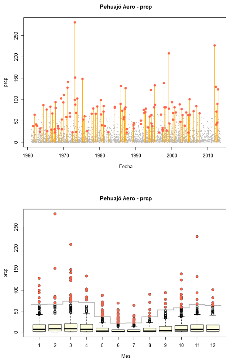
Figura 16. Precipitaciones diarias en Pehuajó, Argentina en 1961-2012. Panel superior: Lluvias diarias (puntos grises) y datos sospechosos (puntos rojos con líneas naranjas). Panel inferior: boxplots mensuales de precipitación diaria (1961-2012) y datos sospechosos (puntos rojos). La línea horizontal gris indica el umbral utilizado en cada mes para definir valores sospechosos. En ambos paneles se utilizan los valores diarios de precipitación \geq 0.1 mm (el umbral que indica un día lluvioso).
