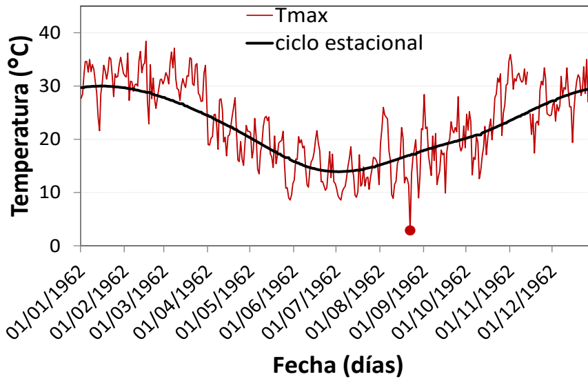
Figura 8. Temperatura máxima diaria observada en Pehuajó (línea roja) y ciclo estacional estimado (línea negra) para el año 1962. El valor de Tmax para el 22 de agosto de 1962 (2.9 °C) está resaltado con un punto rojo, indicando que el control lo identifica como sospechoso.
