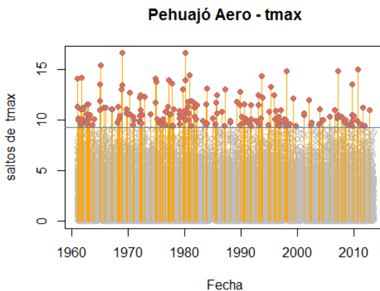
Figura 20. Diferencias absolutas de temperatura máxima en dos días consecutivos en Pehuajó, Argentina, en 1961-2012. La línea horizontal azul indica el percentil 0.99, utilizado para la identificación de saltos extremos. Los puntos rojos unidos al origen del eje x por líneas anaranjadas indican saltos extremos.
