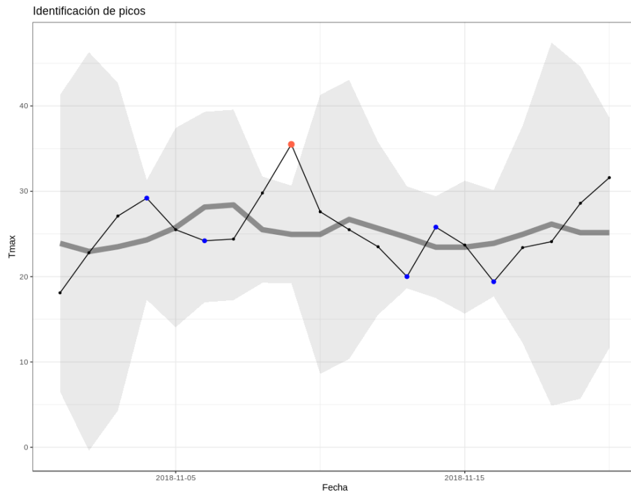
Figura 24. Ejemplos de la detección de picos extremos en las estaciones meteorológicas Pehuajó, Argentina (panel A) y Londrina, Brasil (panel B). La línea fina negra indica la serie temporal de temperatura máxima diaria para una parte del registro en cada estación. La línea gris más gruesa representa la mediana de los valores dentro de ventanas móviles de 7 días. El área gris representa la zona entre el umbral superior e inferior de valores sospechosos (ver descripción del cálculo en el texto). Los días indicados con puntos azules indican picos positivos o negativos de cualquier magnitud. Los puntos rojos son picos de una magnitud sospechosa (se extienden más allá de la zona gris).
