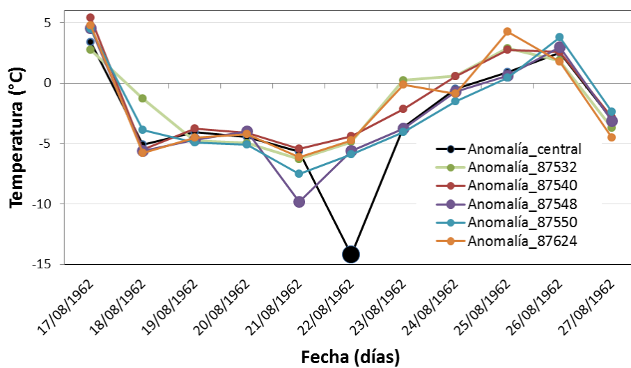
Figura 30. Panel superior: Temperatura máxima observada en la estación central (Pehuajó, Argentina) y cinco estaciones vecinas (General Pico (87532), Trenque Lauquén (87540), Junín (87548), Nueve de Julio (87550) y Anguil (87624)). Las series corresponden al período entre el 17 y el 27 de agosto de 1962. Panel inferior: Diferencias absolutas entre anomalías de temperaturas en la estación central y en estaciones vecinas, 21 al 23 de agosto de 1962. Las anomalías se calculan respecto a un valor promedio estimado para cada estación y día del año. Si todas las diferencias absolutas consideradas están por encima de un umbral determinado (la línea horizontal en la figura) se considera que el valor de la estación central es sospechoso.
