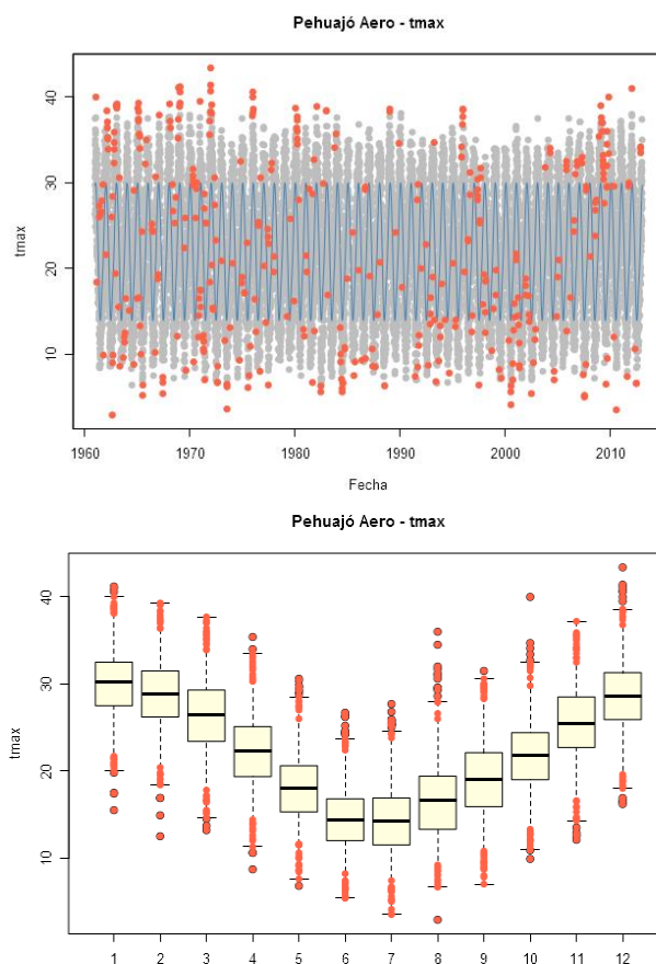
Figura 10. Temperatura máxima diaria en Pehuajó, Argentina, 1961-2012. Panel superior: Ciclo estacional estimado (línea azul), datos (puntos grises) y datos sospechosos (puntos rojos). Panel inferior: boxplots mensuales (1961-2012) y datos sospechosos (puntos rojos).
