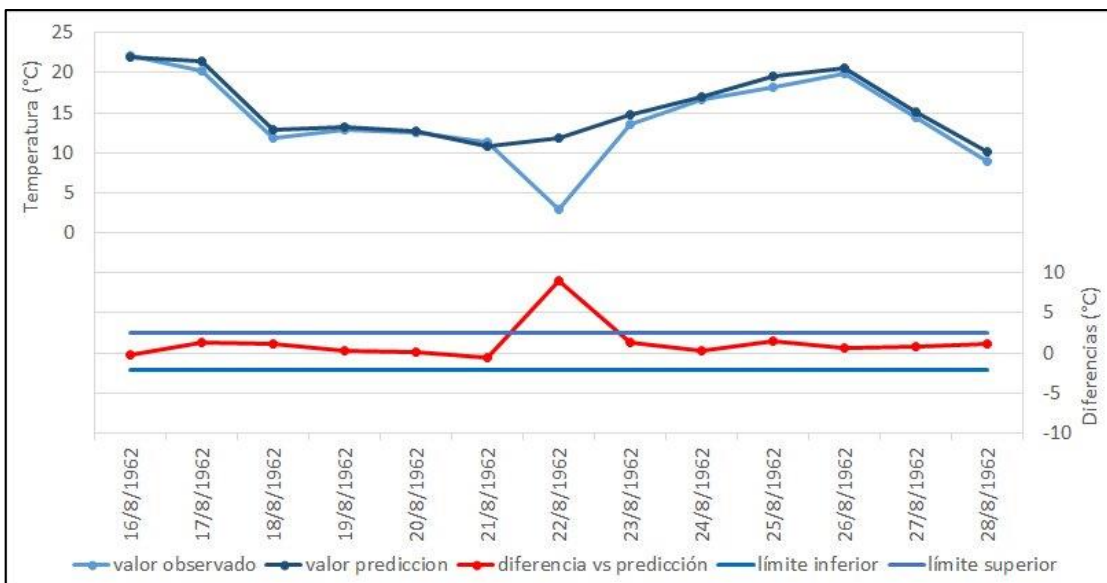
Figura 31. Panel superior: Temperatura máxima observada en la estación central (Pehuajó, Argentina) y valor de la predicción utilizando IDW. Las series corresponden al período entre el 16 y el 28 de agosto de 1962. Panel inferior: diferencias entre el valor de la temperatura máxima y el calculado con IDW, junto con los límites superior e inferior, para los mismos días. Si la diferencia está por fuera de los umbrales determinados se considera que el valor de la estación central es sospechoso.
