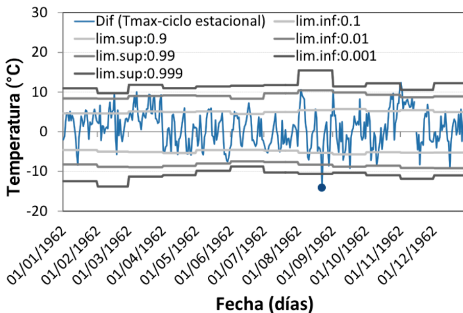
Figura 9. Diferencia entre la temperatura máxima diaria y el ciclo estacional en Pehuajó, año 1962. En tonos de grises se indican los distintos límites del rango aceptable para cada mes según el percentil escogido. El valor sospechoso (punto azul) cae fuera (debajo) del rango más estricto.
