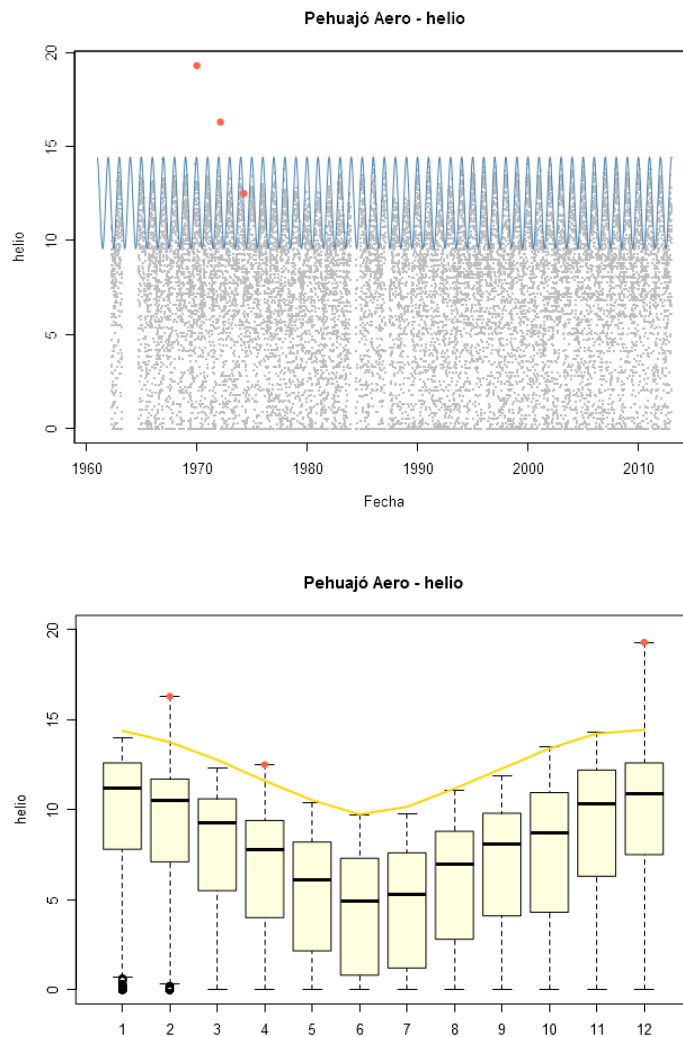
Figura 15. Heliofanía diaria en Pehuajó 1961-2012. Panel superior: Heliofanía máxima teórica para cada día del año (línea azul), valores de heliofanía reportados (puntos grises) y datos sospechosos (puntos rojos). Panel inferior: Boxplots mensuales de heliofanía (1961-2012) y datos sospechosos (puntos rojos). La línea amarilla representa la heliofanía máxima promedio para cada mes.
