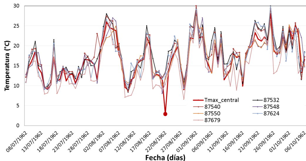
Figura 27. Series observadas de temperatura máxima en la estación central (Pehuajó, Argentina) y seis estaciones vecinas. Las series corresponden a una ventana temporal de 91 días centrada en el 22 de agosto de 1962; la ventana incluye el período entre el 8 de julio y el 6 de octubre de 1962. En general, las trazas de la temperatura máxima observadas en todas las estaciones caen dentro de una banda relativamente estrecha. Una excepción es la observación del 22 de agosto de 1962 en Pehuajó, que es sensiblemente más baja que los registros de ese día en las estaciones vecinas; la estimación ponderada del valor en la estación central (Pehuajó) para el 22 de agosto de 1962 tiene un valor de 12.1 °C y un intervalo de confianza entre 5.03 y 19.17 °C. La observación identificada como sospechosa (2.9 °C) cae fuera del intervalo.
