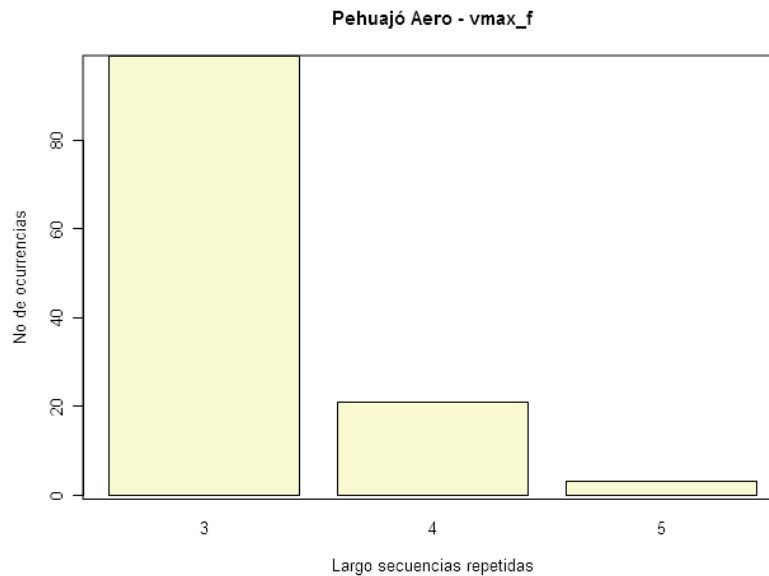
Figura 18. Número de ocurrencias de secuencias con valores de velocidad de viento máximo diario repetidos durante 3, 4 y 5 días en Pehuajó, Argentina. En los datos 1961-2012 no hay secuencias repetidas más largas (> 5 d) que las incluidas en la figura.
