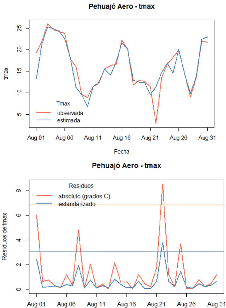
Figura 30. Panel superior: Valor observado de temperatura máxima para una estación central (Pehuajó, Buenos Aires, Argentina) y valor estimado a partir de 4 estaciones vecinas. Las series corresponden a agosto de 1962. Panel inferior: Series temporales de diferencias o residuos entre valores observados y estimados para Pehuajó. Los umbrales considerados para considerar como sospechosos a los residuos absolutos (en °C) y estandarizados (sin unidades) se muestran como líneas horizontales en los colores respectivos. El valor para el 22 de agosto de 1962 muestra residuos por encima de los dos umbrales.
