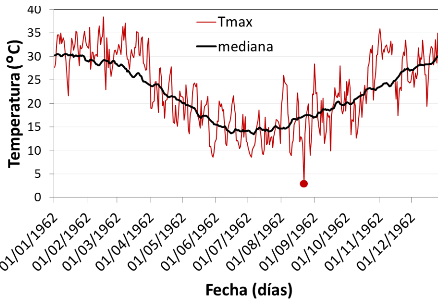
Figura 11. Temperatura máxima diaria observada en Pehuajó (rojo) y mediana de valores para cada día del año (línea negra), año 1962. El valor de Tmax para el día 1962-08-22 (2.9 °C) está indicado con un punto rojo, indicando que el control lo identifica como sospechoso.
