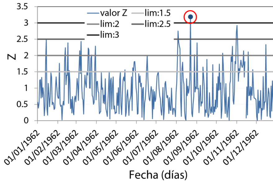
Figura 14. Estadístico Z calculado para cada día del año 1962 en Pehuajó. En tonos de grises se indican los distintos límites del rango aceptable. El valor sospechoso para el día 1962-08-22 cae fuera (encima) del rango más estricto ( Z > 3 ).
