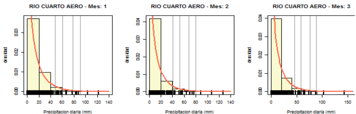
Figura 17. Histogramas de precipitaciones diarias en estación meteorológica Río Cuarto, Córdoba, Argentina. De izquierda a derecha, los histogramas corresponden a los meses de enero, febrero y marzo, respectivamente. La línea naranja en cada panel indica la distribución gamma ajustada a los valores de cada mes. Las líneas verticales grises corresponden a los percentiles 0.950, 0.975, 0.990 y 0.995 respectivamente.
