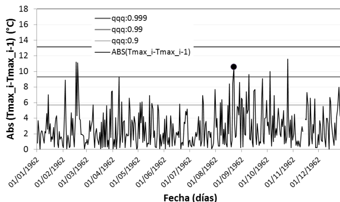
Figura 22. Valor absoluto de las diferencias entre Tmax en dos días consecutivos en Pehuajó para cada día de 1962. Las líneas horizontales indican diferentes umbrales posibles para la identificación de diferencias extremas basados en diferentes percentiles (0.900, 0.990 y 0.999). La diferencia de temperatura entre el 22 y 21 de agosto de 1962 excede el umbral definido por el percentil 0.990; el salto se debe al valor erróneo registrado el 22 de agosto.
