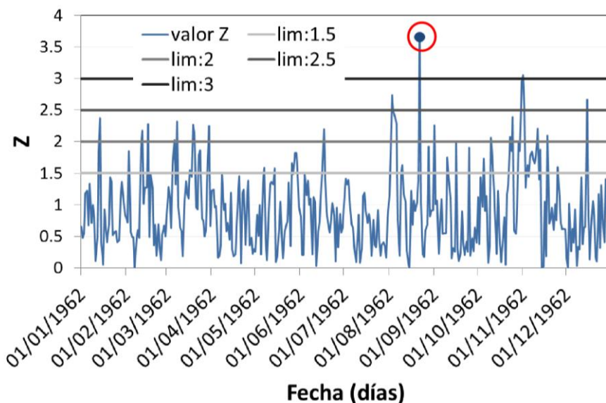
Figura 12. Estadístico Z calculado para cada día del año 1962 en Pehuajó. En tonos de grises se indican los distintos límites del rango aceptable. El valor sospechoso para el día 1962-08-22 (punto azul) cae fuera (encima) del rango más estricto ( z > 3 ).
