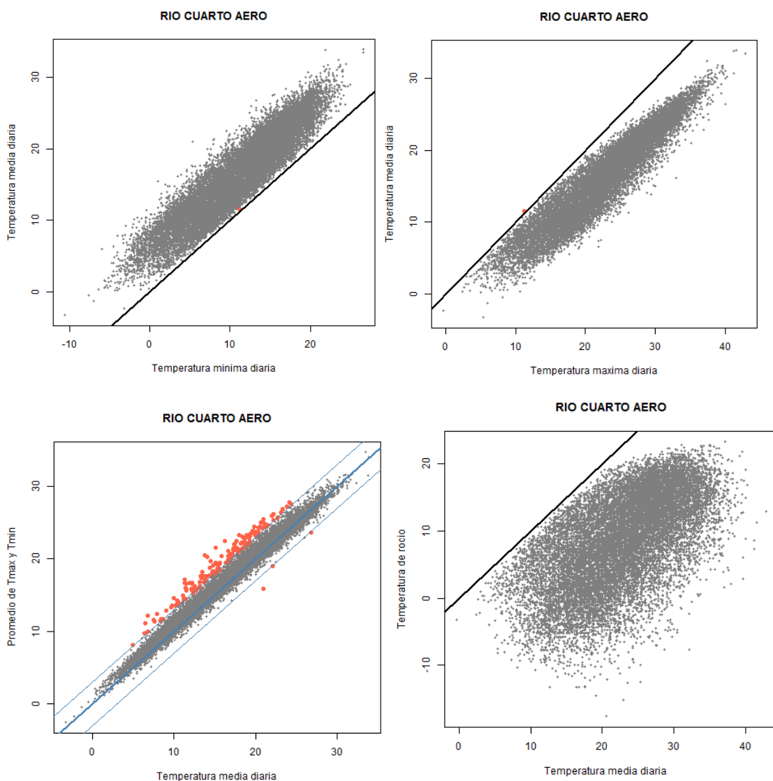
Figura 26. Visualización de los controles de consistencia entre temperaturas diarias. Arriba, izquierda: relación entre temperatura mínima (eje x) y media (eje y). La línea 1:1 se indica en negro; hay un punto (rojo) identificado como sospechoso; aunque este punto está por encima de la línea 1:1 (o sea, T_{med} \geq T_{min} ), se marca el punto porque falla la relación entre T_{med} y T_{max} (ver panel de arriba a la derecha). Arriba, derecha: relación entre temperatura máxima (eje x) y media (eje y); se puede ver un punto rojo en el cual T_{med} > T_{max} . Abajo, izquierda: relación entre temperatura media calculada con varias observaciones diarias (eje x) y la semisuma de temperaturas extremas (eje y). Son puntos sospechosos los que están por encima o por debajo de una tolerancia determinada con respecto a la línea 1:1. Abajo, derecha: relación entre temperatura media (eje x) y temperatura de rocío (eje y).
