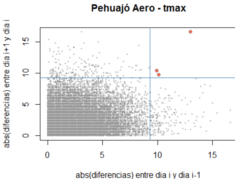
Figura 23. Diferencias absolutas de temperatura máxima entre un día y los días anterior (eje x) y siguiente (eje y) para Pehuajó, 1961-2012. En cada eje se indica el valor del umbral que define diferencias extremas (en este caso, el percentil 0.99). Los puntos para los cuales las dos diferencias de temperatura exceden los dos umbrales (marcados en rojo en el cuadrante superior derecho) se consideran “picos” extremos.
