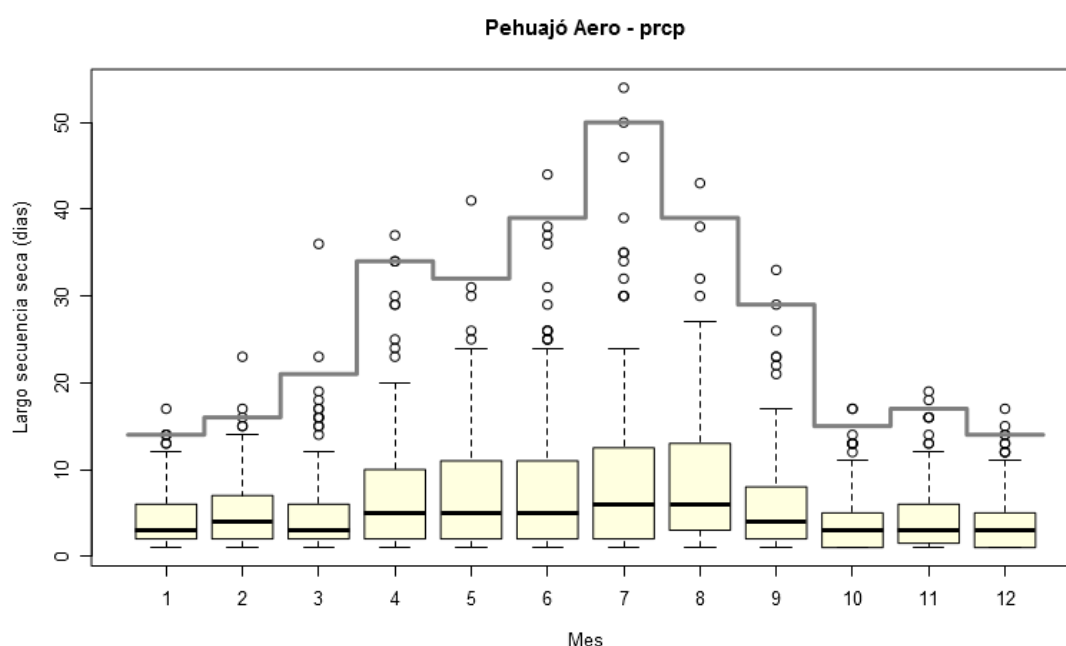
Figura 19. Boxplots de la distribución de extensión de secuencias de días sin precipitación en Pehuajó, Argentina, en el periodo 1961-2012. La línea gris escalonada indica los umbrales para identificación de largos extremos para cada mes (en este caso, el percentil 0.995). Durante los meses con mayor precipitación (por ejemplo, diciembre, enero), el umbral está alrededor de los 14-16 días, mientras que, en los meses más secos, las secuencias secas deben superar los 40 días para ser consideradas extremas.
